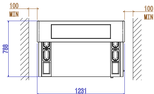
Felülnézet
